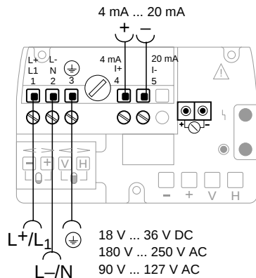
② LUC-T20 4 fils, y compris alimentation
