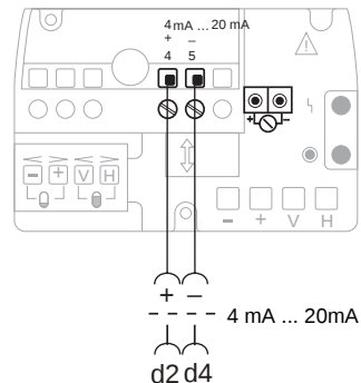
③ LUC-T30 Vierdraht, inklusive Netzversorgung 18 V ... 36 V DC, 180 V ... 250 V AC 90 V ... 127 V AC
