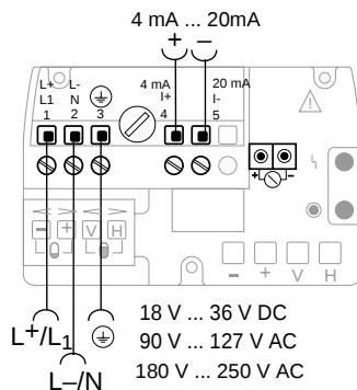
② LUC-T20 Vierdraht, inklusive Netzversorgung
