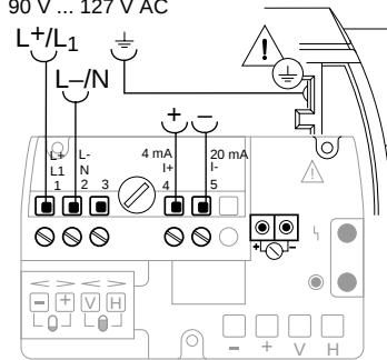
③ LUC-T30 Vierdraht, inklusive Netzversorgung 18 V ... 36 V DC, 180 V ... 250 V AC 90 V ... 127 V AC
