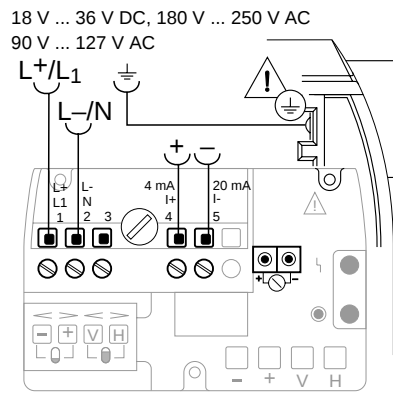
③ LUC-T30 4 fils, y compris alimentation
