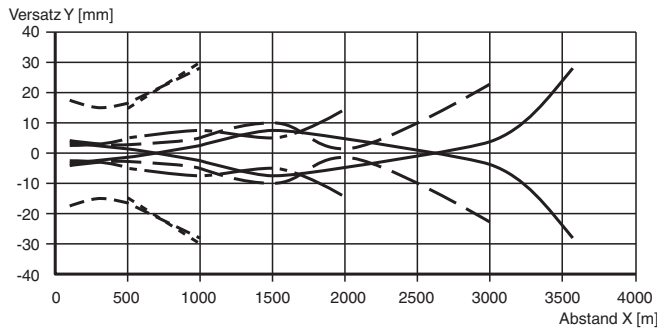
Charakteristische Ansprechkurve
