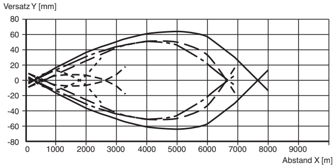
Charakteristische Ansprechkurve
