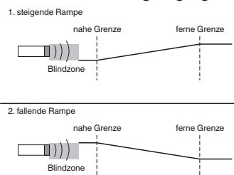
Charakteristische Ansprechkurve
