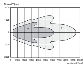
Charakteristische Ansprechkurve
