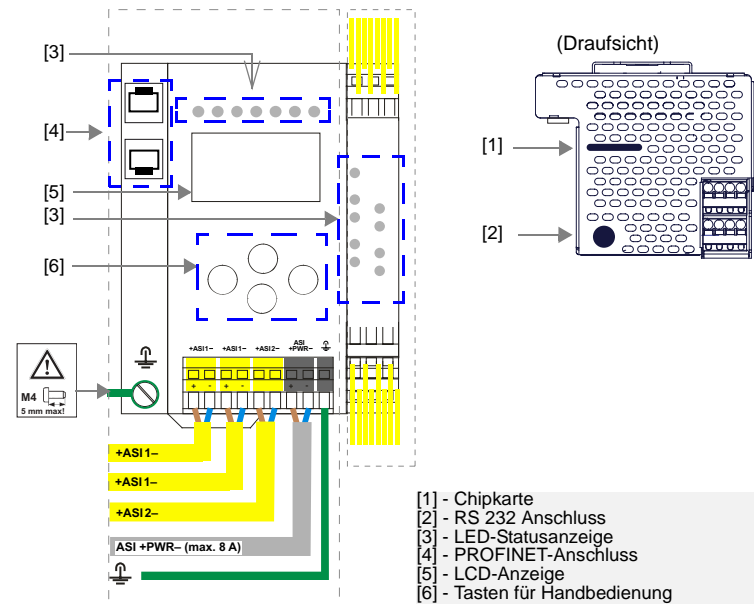
Abb. 1 Anschlussbild Gateway
