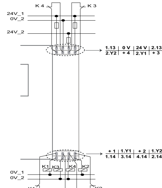
Abb. 2: Anschlussbild Sicherheitseinheit
