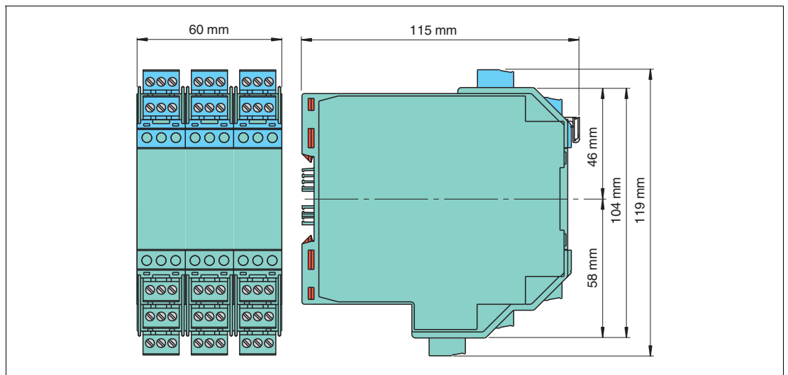
Abbildung 7.6 Abmessungen (B x H x T)
