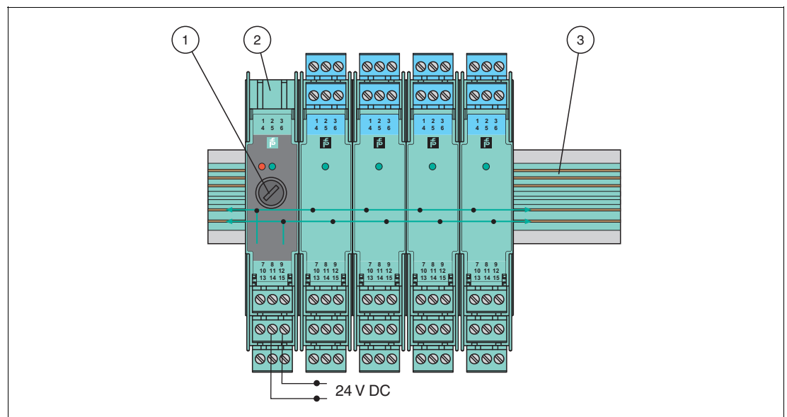
Abbildung 3.8 Power-Rail-Installation
