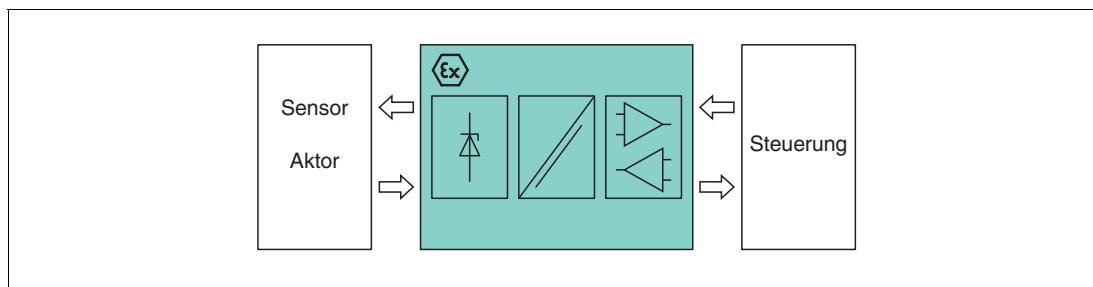
Abbildung 2.1 Funktion – Signale trennen, verstärken und umformen
