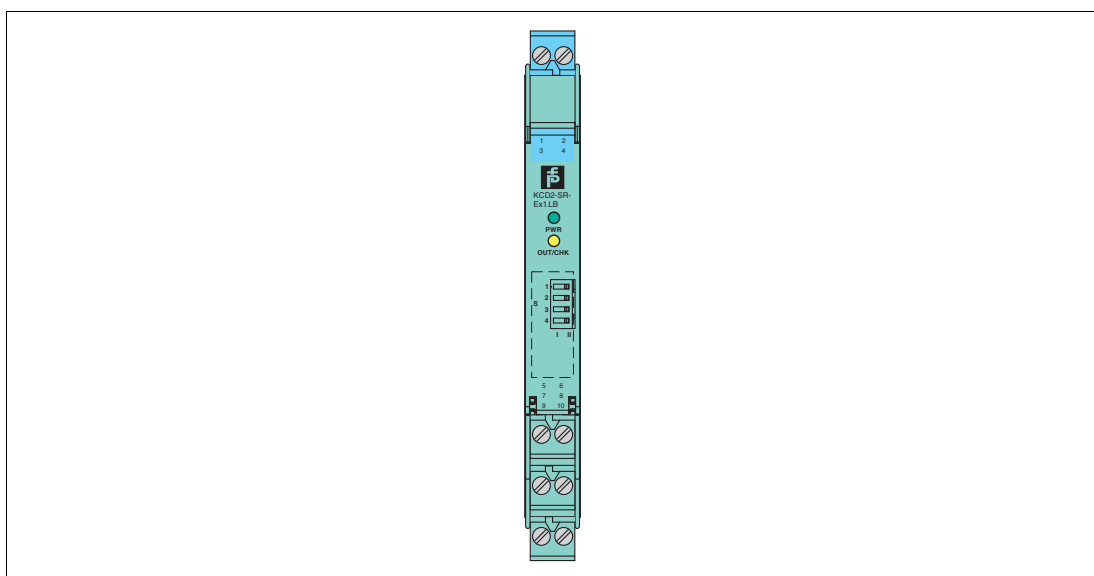
Abbildung 2.3 Gehäuse KC-Geräte (12,5 mm)
