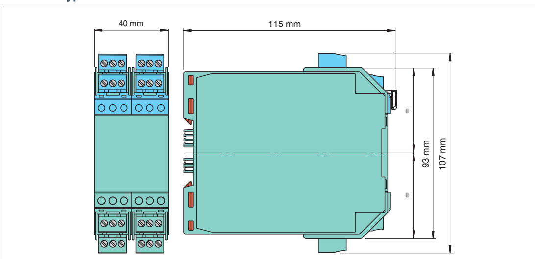
Abbildung 7.4 Abmessungen (B x H x T)
