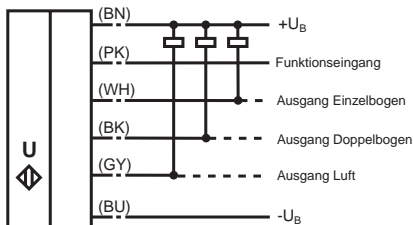
Bild 7.1: Elektrischer Anschluss
