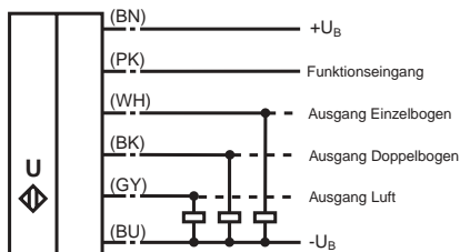
Bild 7.1: Elektrischer Anschluss
