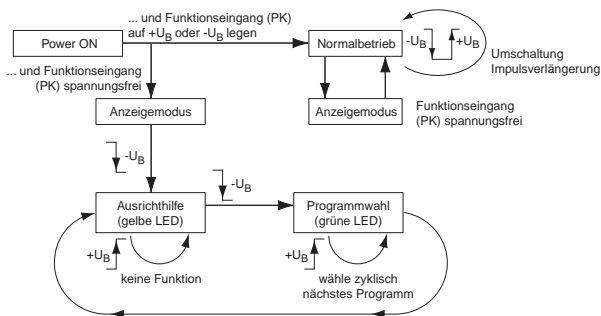
Bild 6.1: Parametrierung
