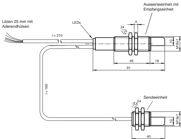
Bild 7.2: Abmessungen
