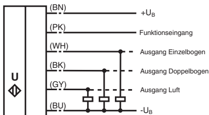
Bild 7.1: Elektrischer Anschluss
