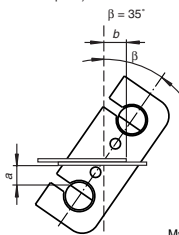
Bild 5.1: empfohlene Winkeleinstellungen
