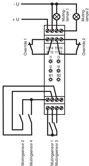
Abbildung 7.11: Anschlussbeschriftung Muting-Modul
