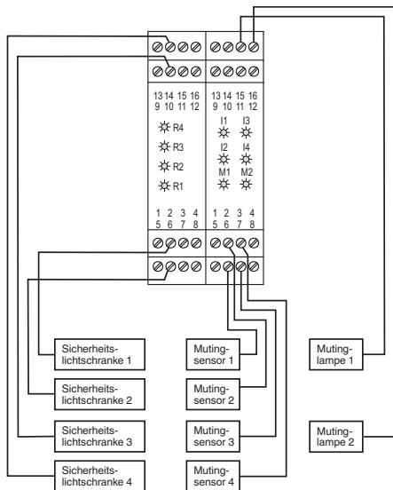
Abbildung 7.9: Doppelmuting schematische Anschlussbelegung der Module
