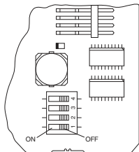
Abbildung 7.2: Lage DIP-Schalter
