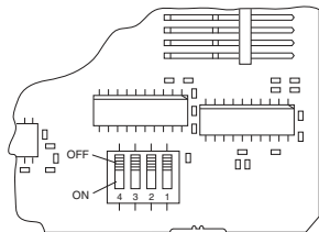
Abbildung 7.18: Lage DIP-Schalter Sensor-Modul
