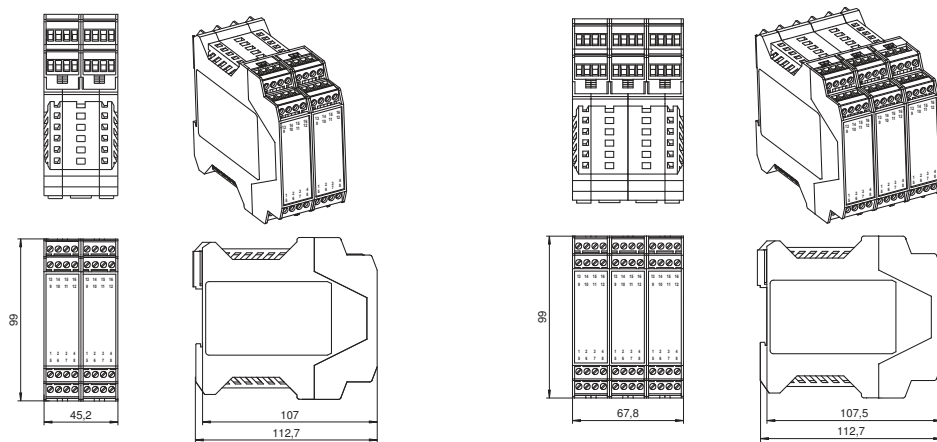
Abbildung 13.2: Abmessungen SB4-OR-4CP und SB4-OR-4CP-4C (SB4-OR-4CP-4M)
