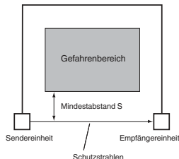
Abbildung 8.1: Mindestabstand zwischen BWS und Gefahrenbereich
