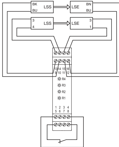
Abbildung 7.15: Anschlussbeispiel 4-kanaliges Sensor-Modul
