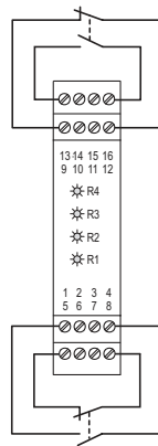
Abbildung 7.17: Anschluss zweier 2-kanaliger, antivalenter Sicherheitseinrichtungen an ein 4-kanaliges Sensor-Modul
