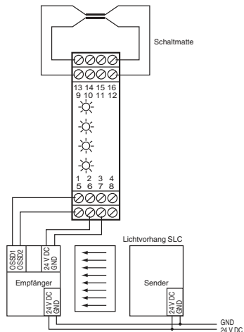
Abbildung 7.22: Anschluss eines Sicherheitslichtvorhangs SLC und einer Schaltmatte an ein 4X-Modul
