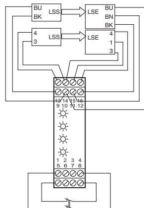
Abbildung 7.21: Anschlussbeispiel 4-kanaliges Sensor-Modul 4X
