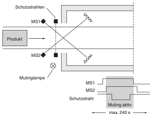
Abbildung 6.3:zeitfensterbegrenztes Muting
