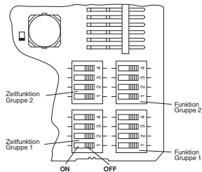
Abbildung 7.7: Lage DIP-Schalter
