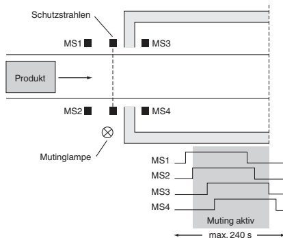
Abbildung 6.1:paralleles Muting
