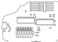
Abbildung 7.24: Lage DIP-Schalter Sensor-Modul 4X(P)
