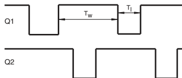
Abbildung 7.19: Zeitdiagramm Testimpulse
