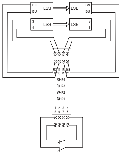
Abbildung 7.16: Anschluss zweier Lichtschranken und einer 2-kanaligen Sicherheitseinrichtung an ein 4-kanaliges Sensor-Modul
