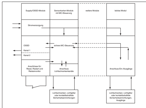
Abbildung 5.1: Geräteaufbau, schematisch
