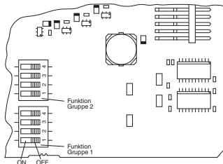
Abbildung 7.12: Lage DIP-Schalter
