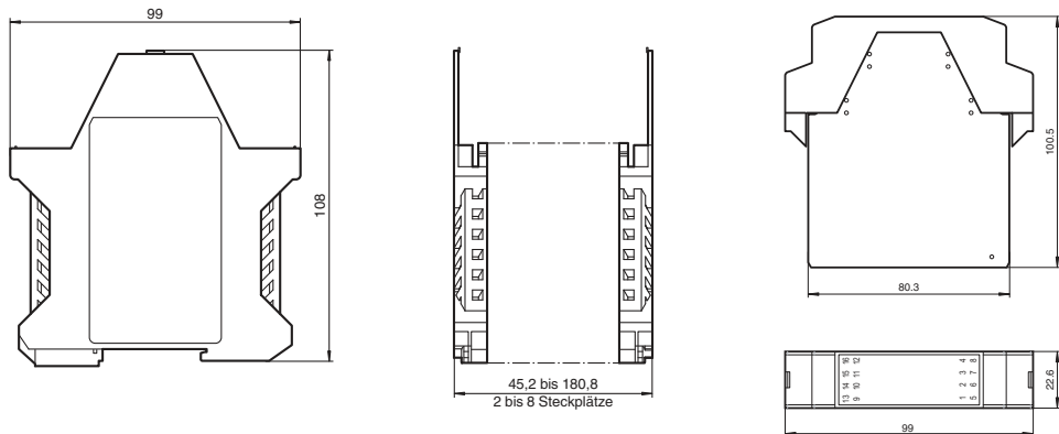
Abbildung 13.1: Abmessungen SB4 Housing und SB4 Module
