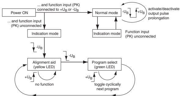
Fig. 5.1: Parameter assignment
