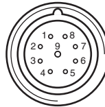
socket
