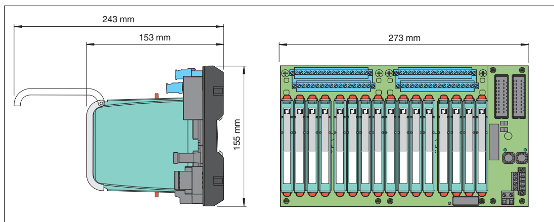
Abbildung 3.2 Abmessungen (B x H x T): 273 x 155 x 153 mm, Tiefe inklusive Modulbestückung
