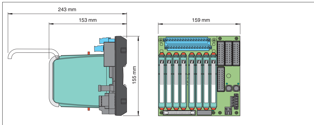
Abbildung 3.1 Abmessungen (B x H x T): 159 x 155 x 153 mm, Tiefe inklusive Modulbestückung
