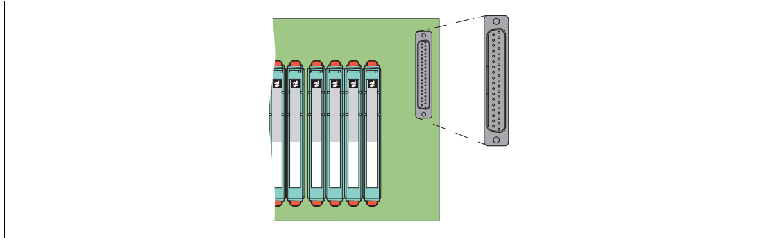
Abbildung 2.5 Sub-D-Stecker, 37-polig, empfohlenes Kabel: CAB-HON-**-S37C32-MX-01000
