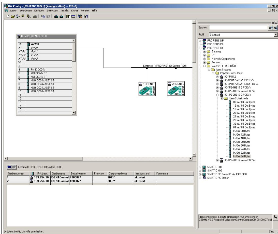
Abbildung 7.2 HW Konfig / Siemens Step7
