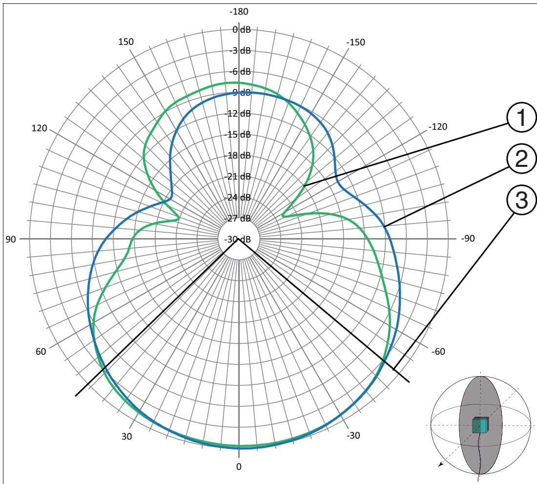
Abbildung 9.3 1 - horizontale Polarisation 2 - vertikale Polarisation 3 - Halbwertsbreite
