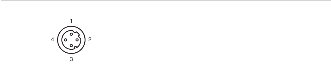
Abbildung 4.3 Anschlussbelegung Ethernet
