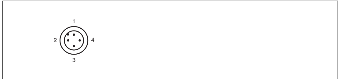
Abbildung 4.2 Anschlussbelegung Spannungsversorgung
