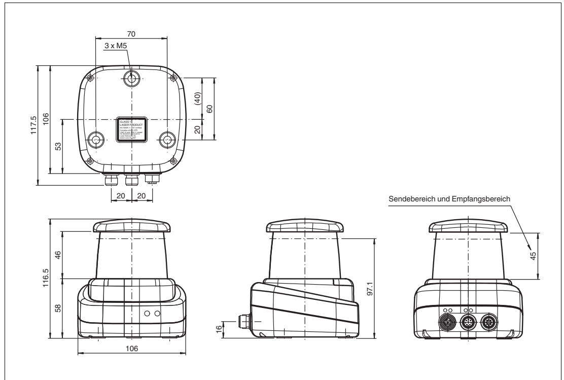
Abbildung 5.1 Abmessungszeichnung R2000
