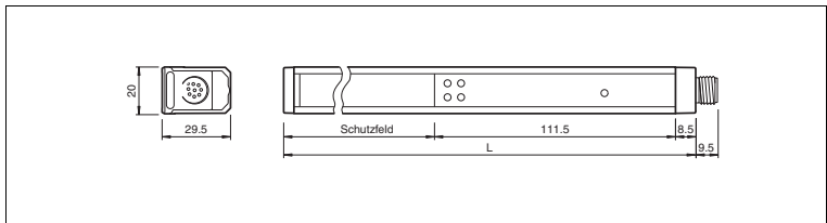
Abbildung 8.2 Abmessungen des Sicherheitslichtvorhangs mit Schutzfeldhöhe \leq 1200 mm
