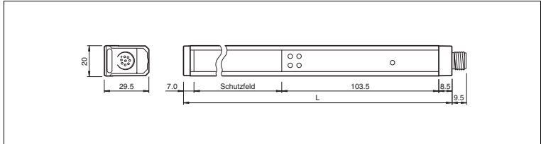
Abbildung 8.1 Abmessungen des Sicherheitslichtvorhangs mit Schutzfeldhöhe von \leq 1200 mm bzw. \leq 2400 mm
