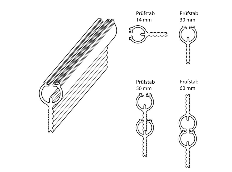
Abbildung 8.7 Prüfstab TR 14/30/50/60
