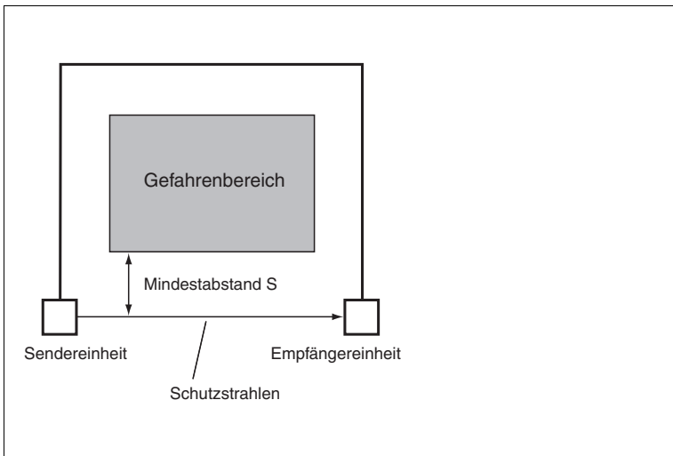
Abbildung 4.1 Erläuterung zum Sicherheitsabstand
