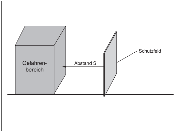
Abbildung 4.2 Erläuterung zum Sicherheitsabstand bei senkrechter Anordnung des Schutzfeldes
