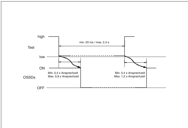
Abbildung 4.5 Zeitlicher Verlauf der OSSD-Schaltzustände beim Auslösen eines Test oder Reset
