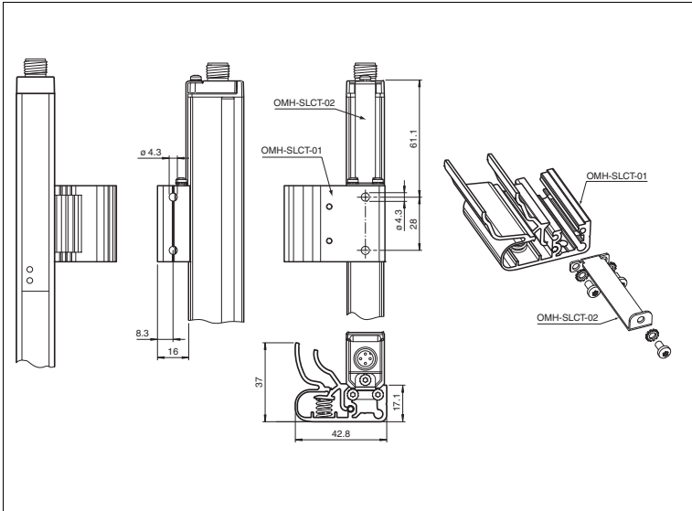
Abbildung 8.4 Abmessungszeichnung und Montage der Montagehilfe OMH-SLCT-01 und OMH-SLCT-02
