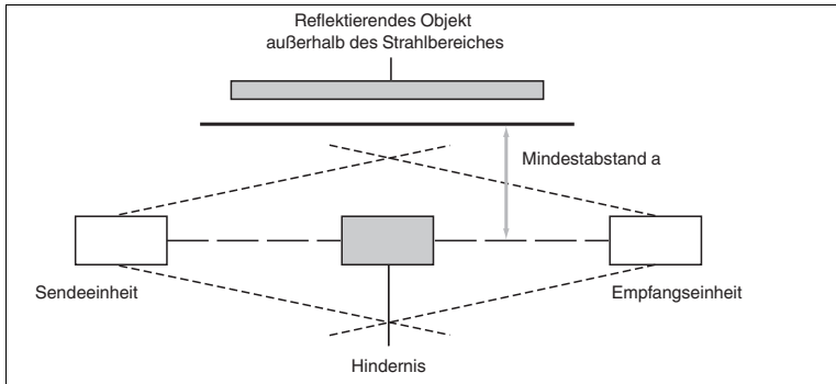
Abbildung 4.4 Erläuterung zur Gefahr der Umspiegelung von Schutzstrahlen
