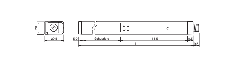
Abbildung 8.3 Abmessungen des Sicherheitslichtvorhangs \geq 1300 mm
