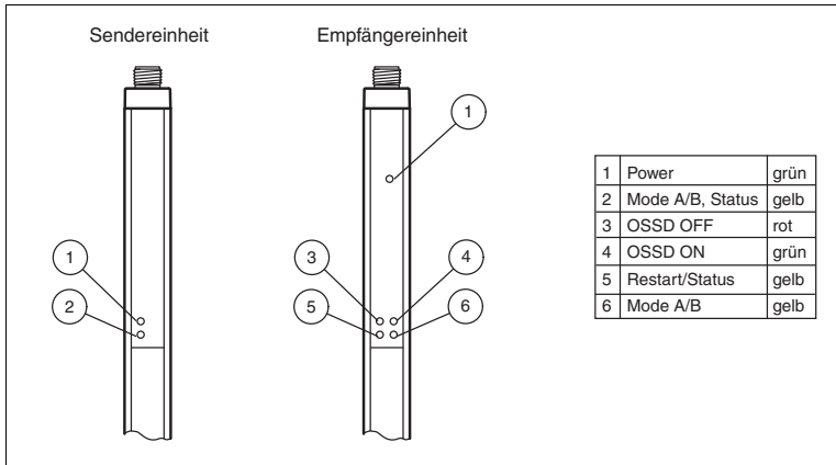
Abbildung 3.2 Anzeigen an der Sender- und Empfängereinheit
