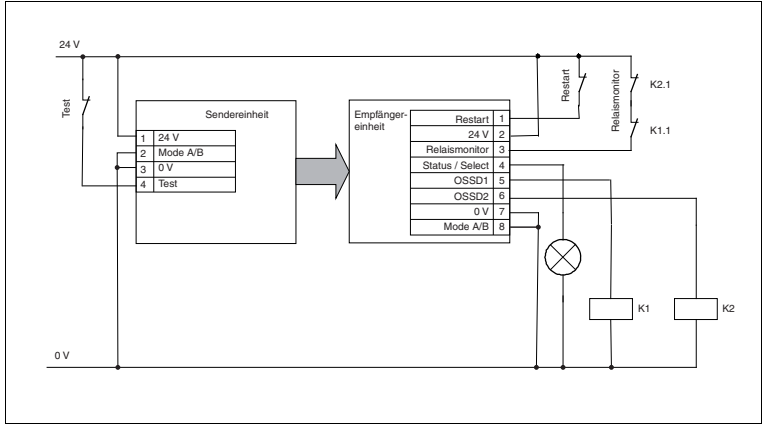
Abbildung 4.6 Anschlussbeispiel mit Restart und Relaismonitor im Mode A
