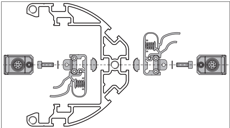
Abbildung 8.5 Beispielmontage einer Montagehilfe OMH-SLCT-01 an eine Montagehalterung
