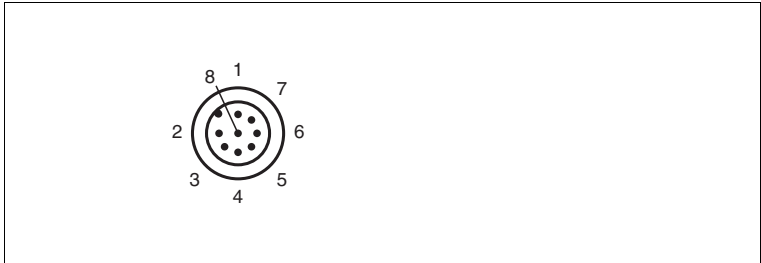
Abbildung 3.4 Anschlussbelegung Empfängereinheit
