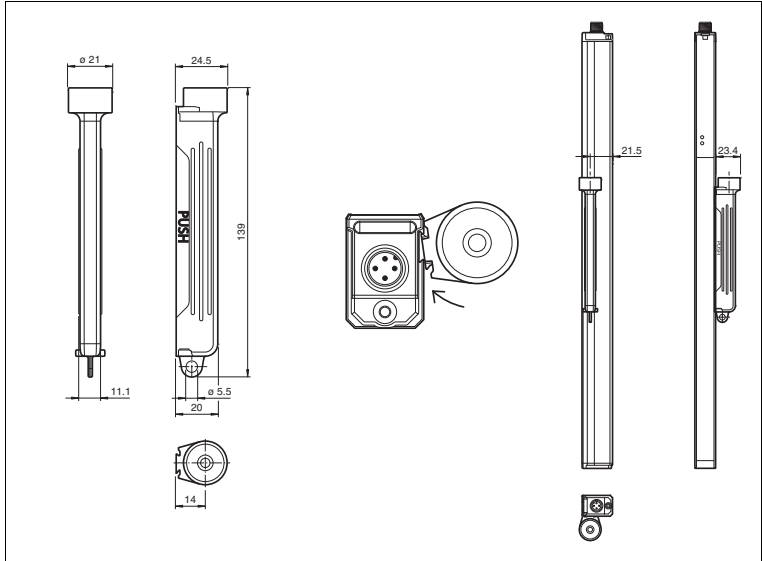
Abbildung 8.6 Abmessungszeichnung und Montage der Ausrichthilfe AA-SLCT-01
