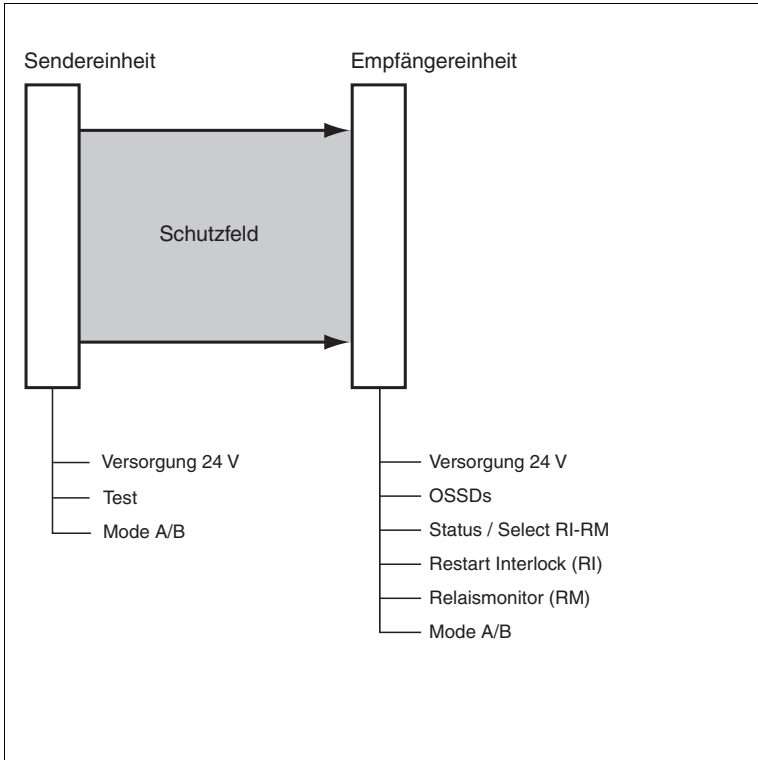
Abbildung 3.1 Schematischer Aufbau einer Schutzfeldeinrichtung
