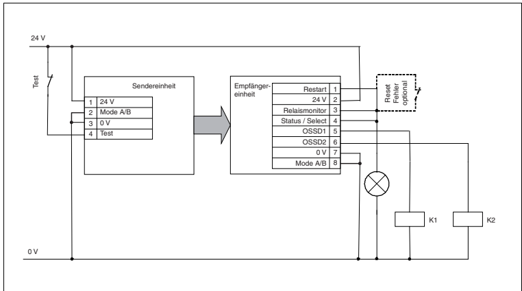
Abbildung 4.7 Anschlussbeispiel ohne Restart und ohne Relaismonitor im Mode A
