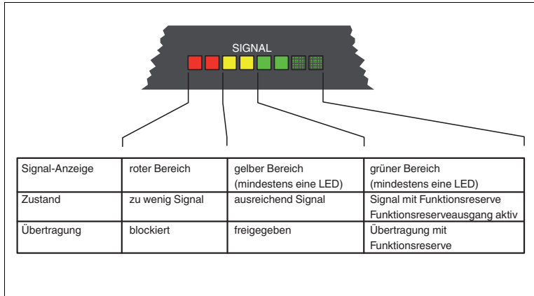
Abbildung 6.2 Zusammenhang von Bargraph-Anzeige und Betriebszustand
