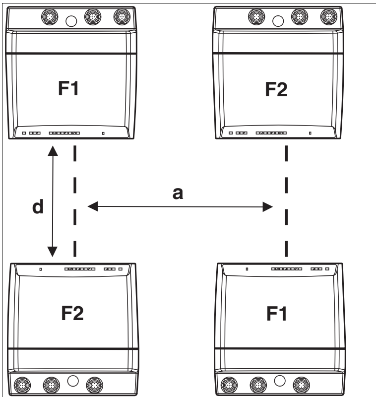
Abbildung 6.7 Parallele Lichtstrecken
