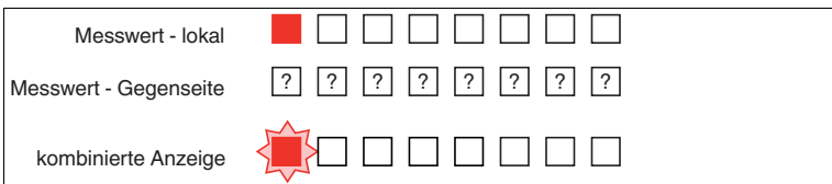
Abbildung 6.6 Der Empfangspegel der Gegenseite ist unbekannt (Unterbrechung des Lichtstrahls, schlecht ausgerichtet etc.). Der Empfangspegel des lokalen Geräts ist klein: rote LED blinkt
