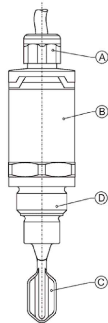
Vibracon mit Kabelschwanz-Version
