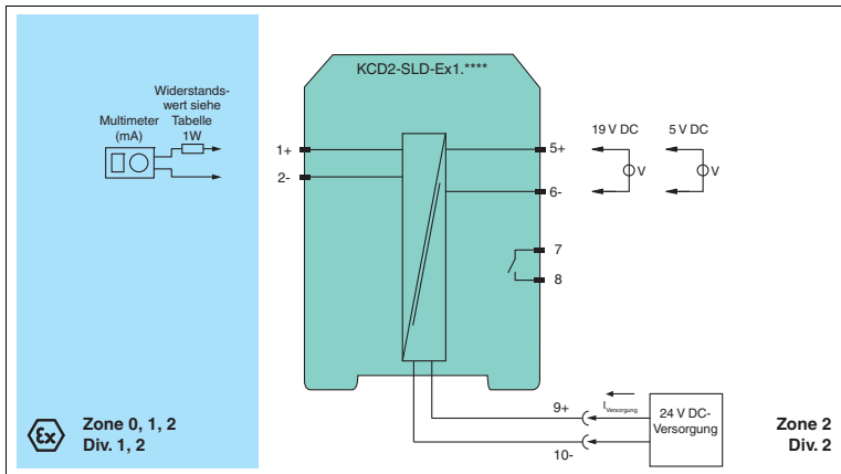
Abbildung 5.1 Aufbau Wiederholungsprüfung für KCD2-SLD-Ex1.***
