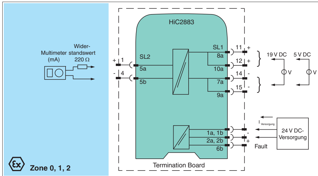
Abbildung 5.1 Aufbau Wiederholungsprüfung für HiC2883
