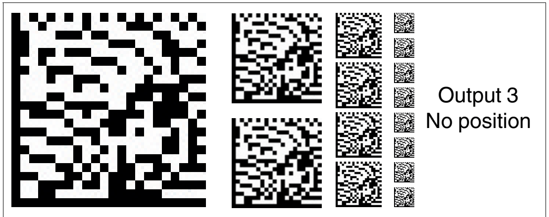
Abbildung 6.22 Der Eingang/Ausgang 3 ist als Ausgang definiert. Dieser Ausgang führt das Potenzial +U_B , solange der Lesekopf keine Positionsinformation liest.
