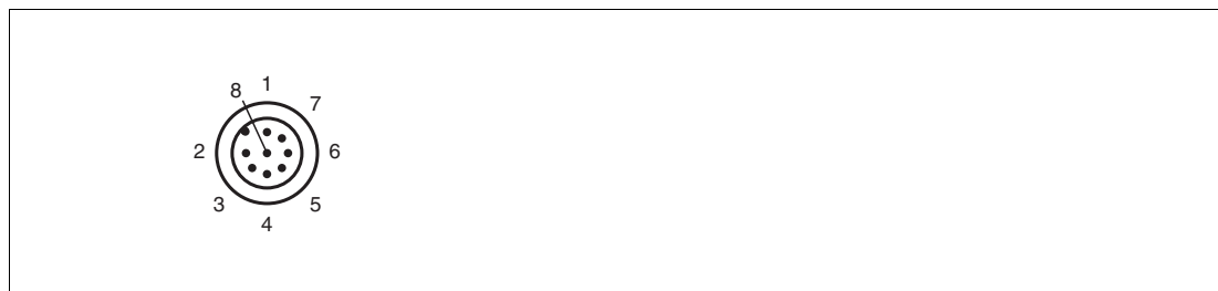
Abbildung 3.5 Steckerbelegung
