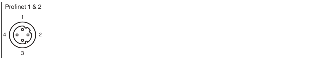
Abbildung 3.4 Steckerbelegung PROFINET
