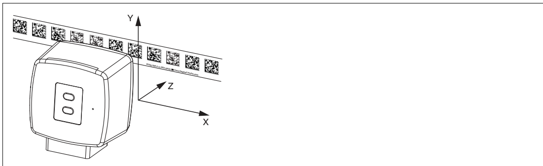
Abbildung 2.1 Schematische Darstellung Orientierung des Codebands und des Lesekopfs
