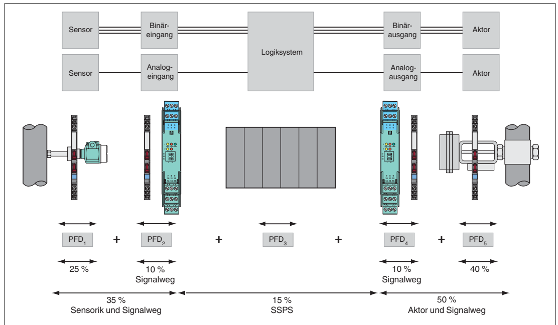
Abbildung 7.1 Beispiel eines vollständigen Sicherheitskreises mit zugeordneten Überspannungsschutz-Barrieren
