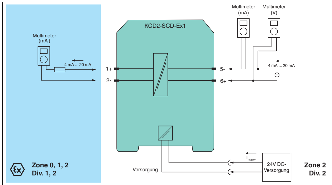
Abbildung 5.1 Aufbau Wiederholungsprüfung für KCD2-SCD-(Ex)1(.SP)
