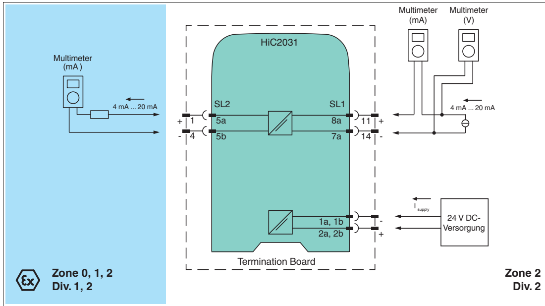
Abbildung 5.2 Aufbau Wiederholungsprüfung für HiC2031
