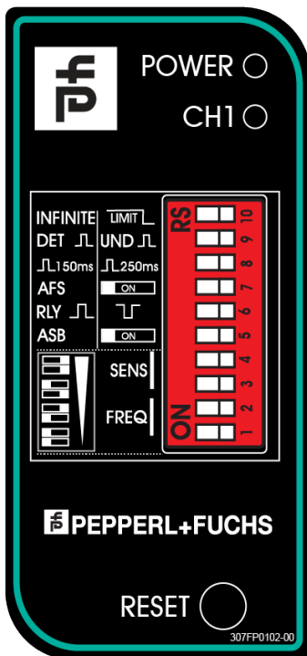
Bild 2. LC20-1 Frontansicht
