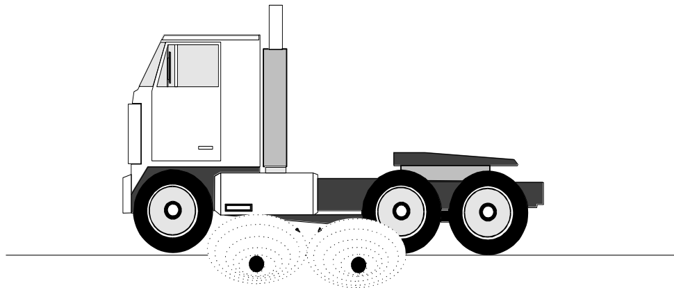
Bild 3. Magnetisches Feld von induktiven Schleifen im Zusammenwirken mit einem Fahrzeug
