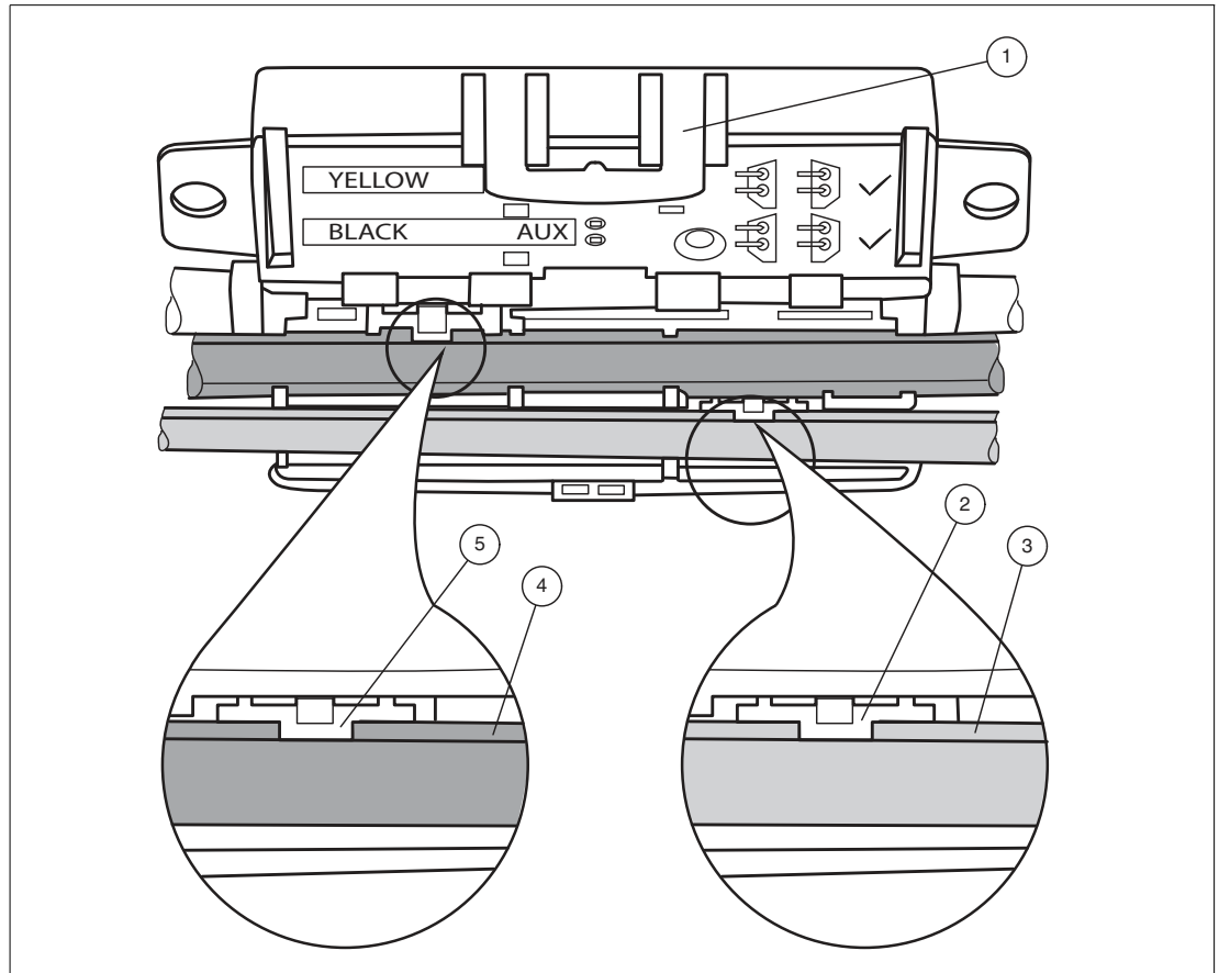
Abbildung 4.1 Anschließen von Flachkabeln auf der Schmalseite
