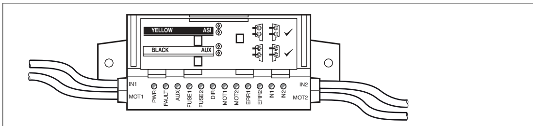
Abbildung 3.3 Statusanzeigen am Motorsteuermodul
