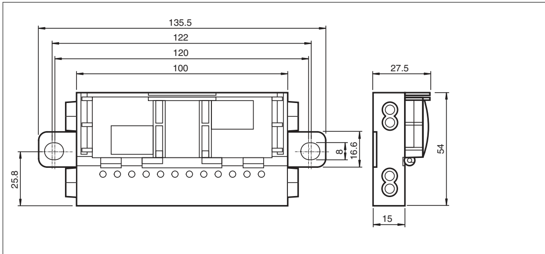
Abbildung 3.2 Gehäuseabmessungen
