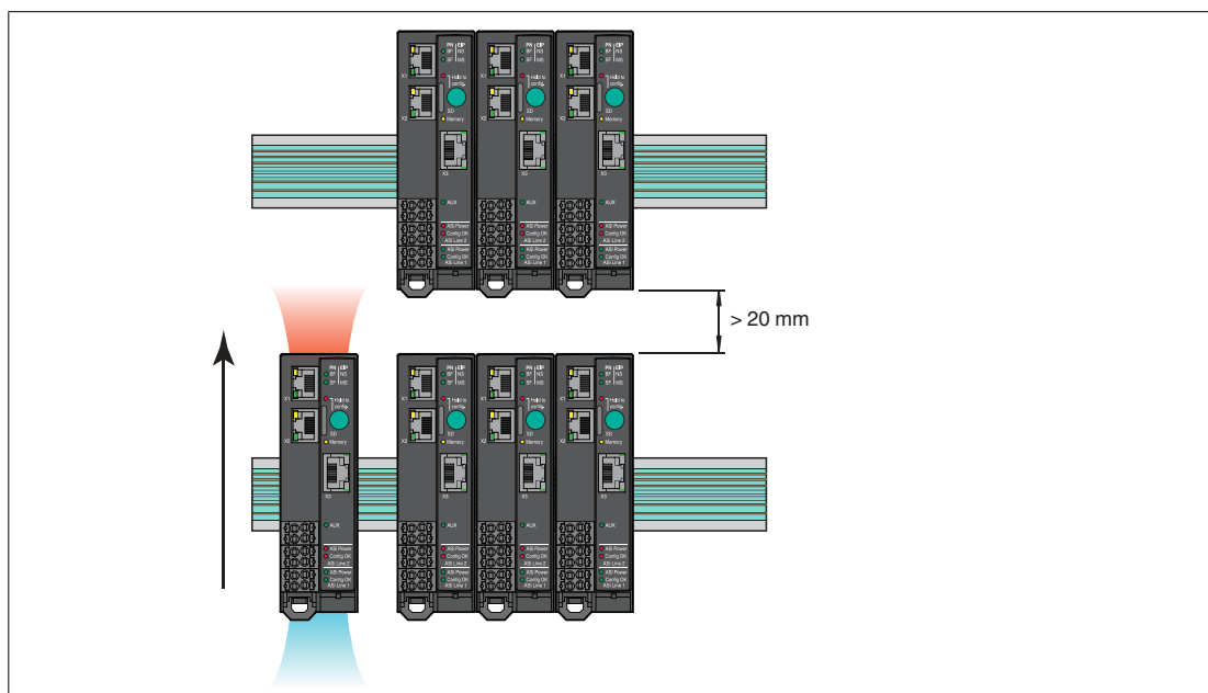
Abbildung 4.8 Mindestabstände
