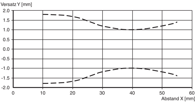
Charakteristische Ansprechkurve
