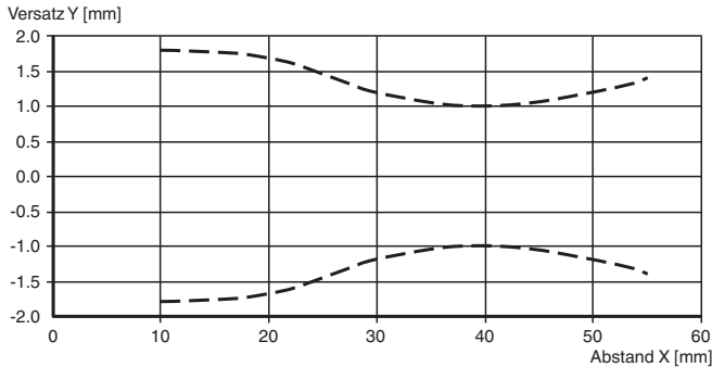
Charakteristische Ansprechkurve
