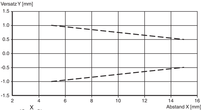
Charakteristische Ansprechkurve
