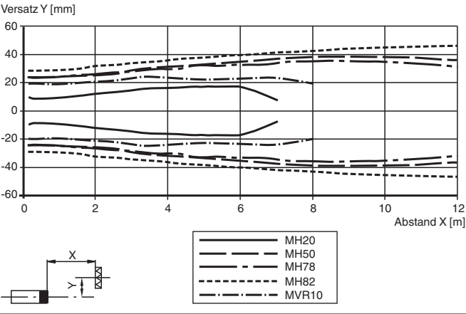
Charakteristische Ansprechkurve
