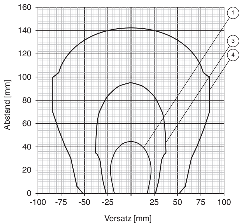
Lesebereich in Luft IQC33-50
