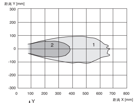
曲线1：平板 100 mm x 100 mm 曲线2：圆棒 Ø 25 mm
