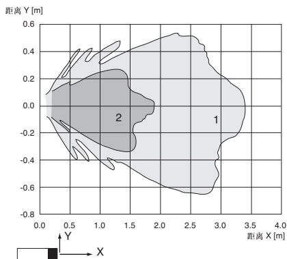
曲线1：平板 100 mm x 100 mm 曲线2：圆棒 Ø 25 mm
