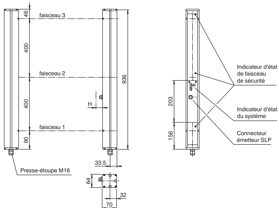
Émetteur SLP...-3-T
