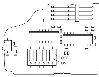
Posición de conmutadores DIP
