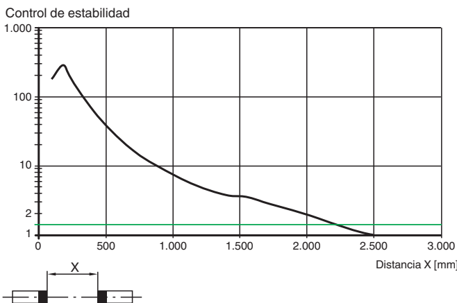
Curva de respuesta característica (modo de alta precisión)
