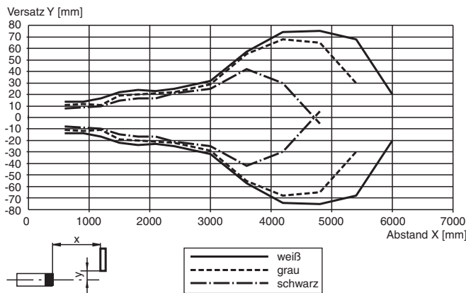
Charakteristische Ansprechkurve (mit Hintergrundausbldung) LT(K)2-8-HS-6000
