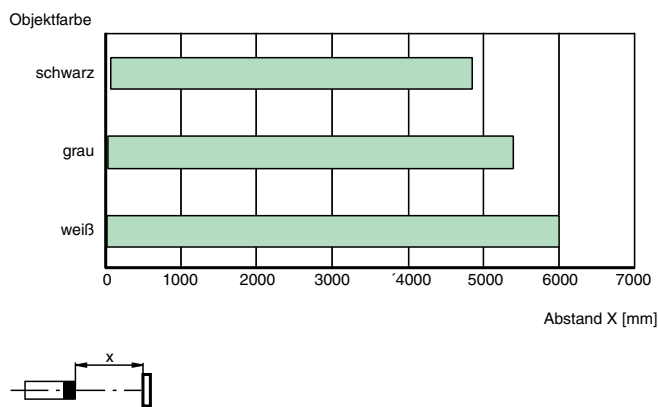
Tastbereiche mit Hintergrundausbldung LT(K)2-8-HS-6000
