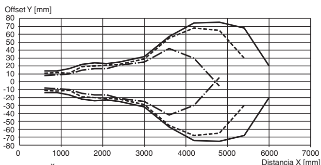
Curva de respuesta característica (con supresión de fondo) LT(K)2-8-HS-6000
