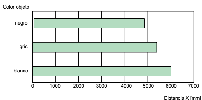
Rangos de detección con upresión de fondo LT(K)2-8-HS-6000
