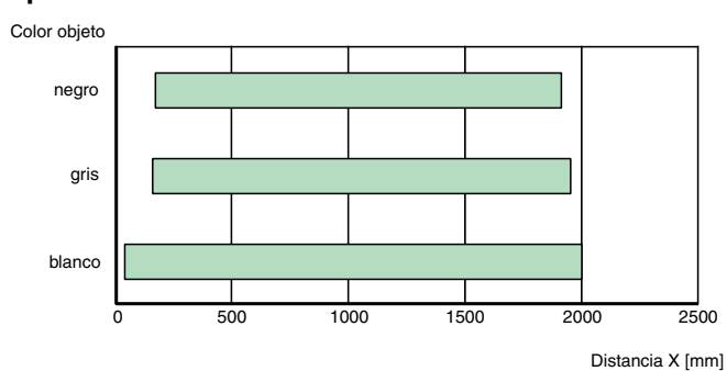
Rangos de detección con upresión de fondo LT(K)2-8-HS-2000
