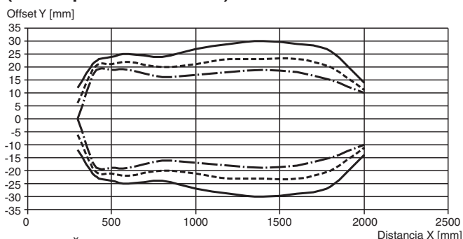
Curva de respuesta característica (con supresión de fondo) LT(K)2-8-HS-2000
