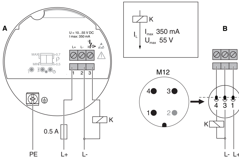
3-Draht DC-PNP, Elektronikereinsatz FEL42 (Beispiel)
