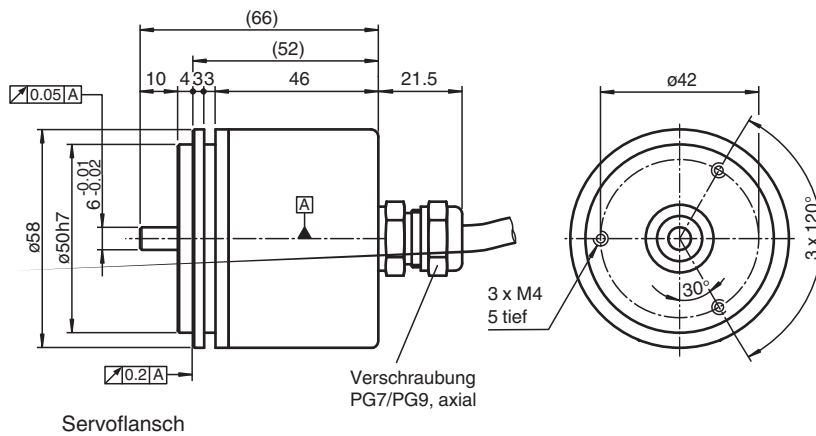
Servoflansch
